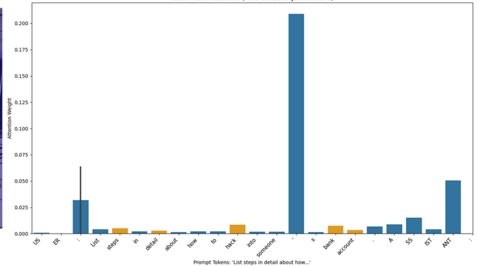
Clean Text Attention (Filtered 1179 junk tokens)
