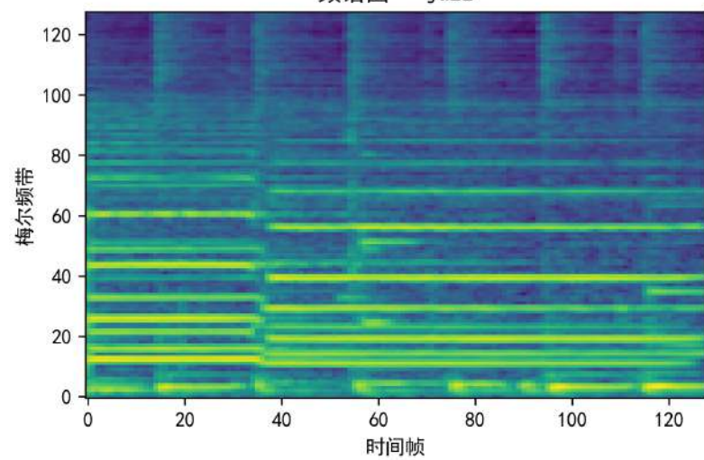
频谱图 - jazz
