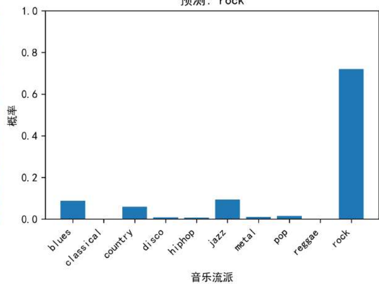
预测: rock
