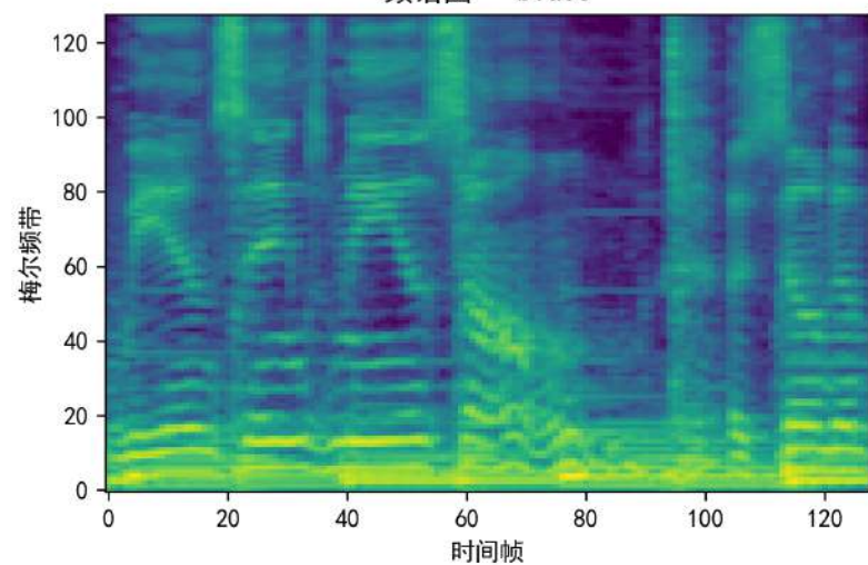
频谱图 - blues
