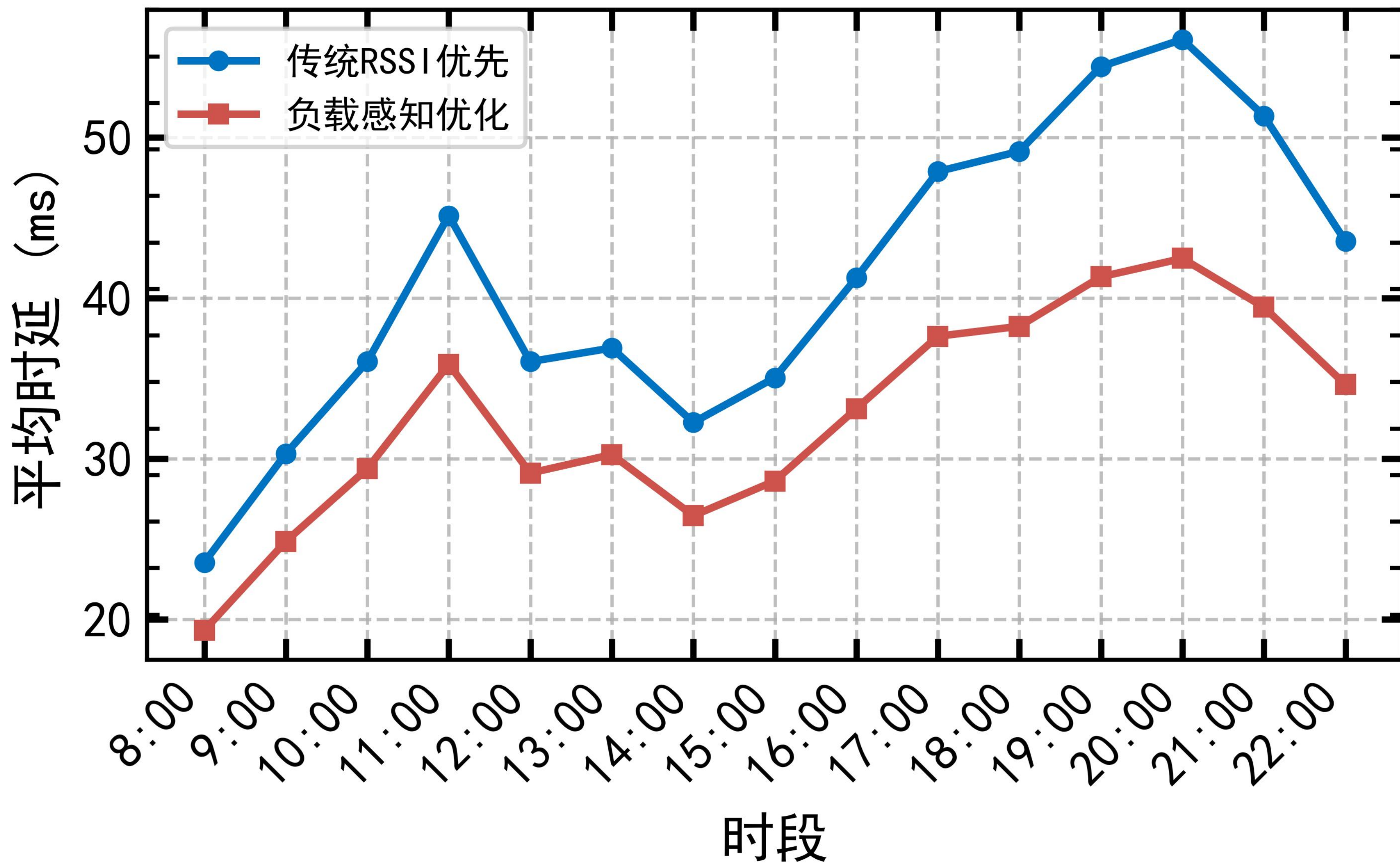
平均时延对比
