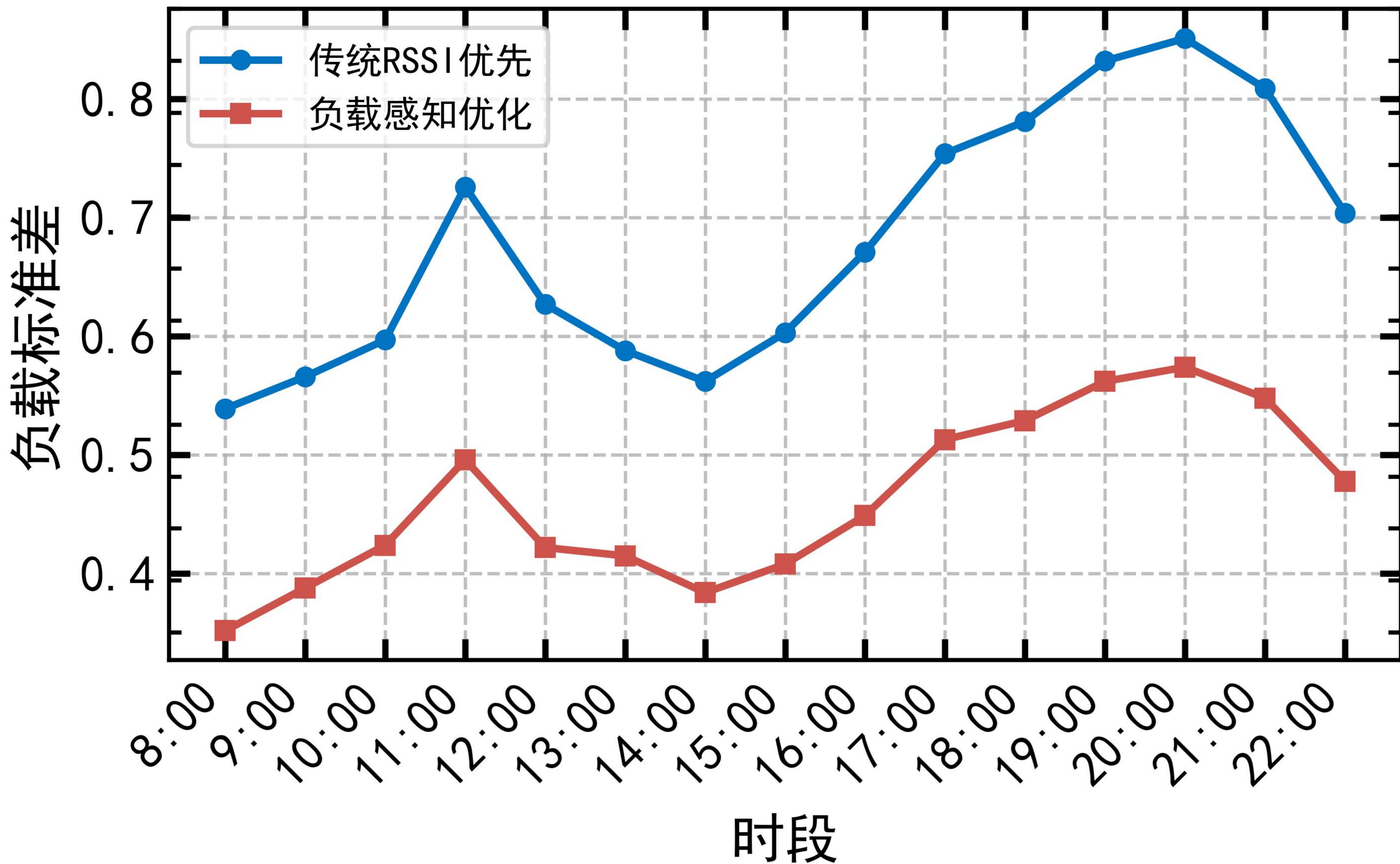
接入点负载标准差对比
