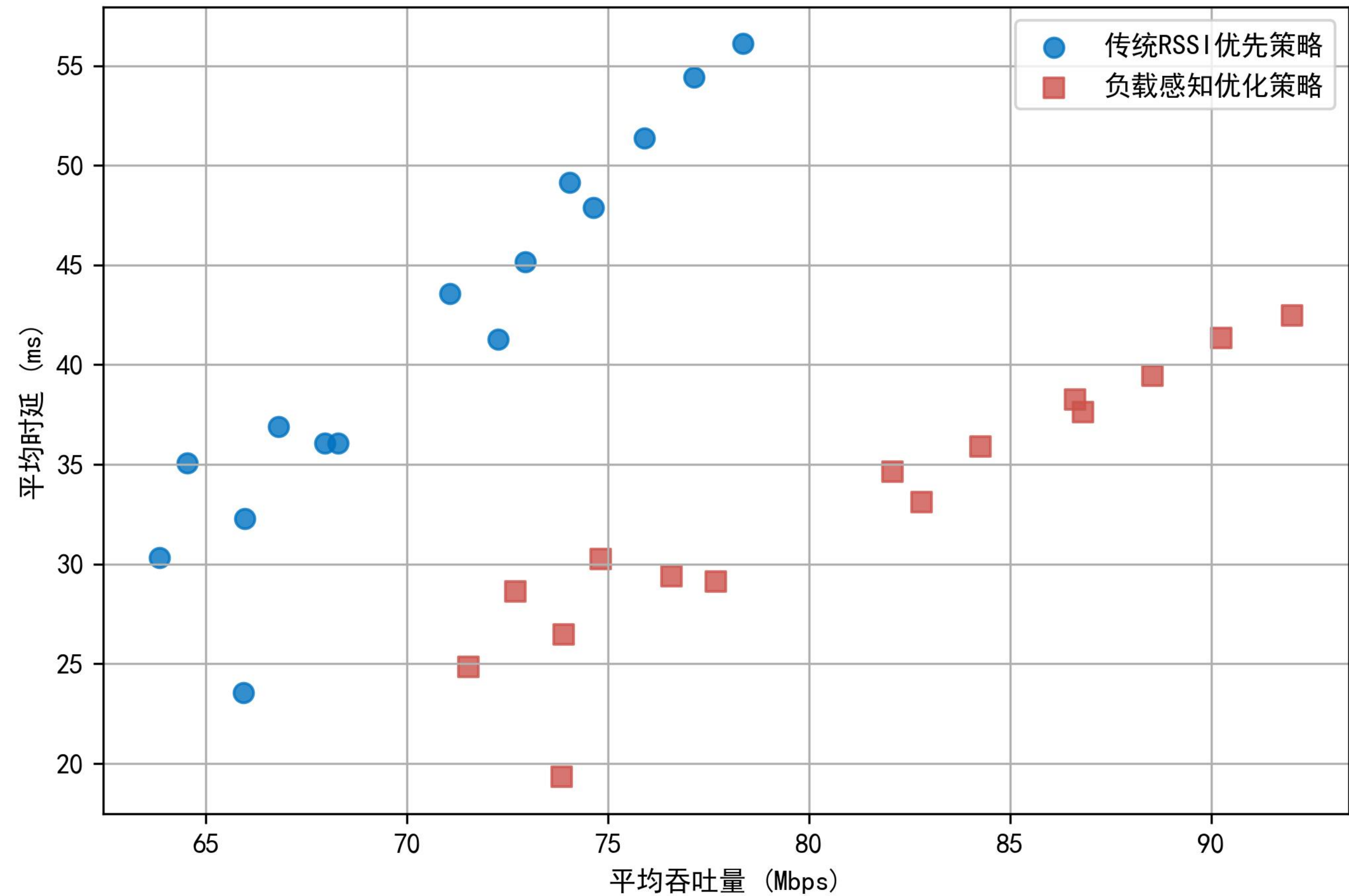
吞吐量与时延关系散点图
