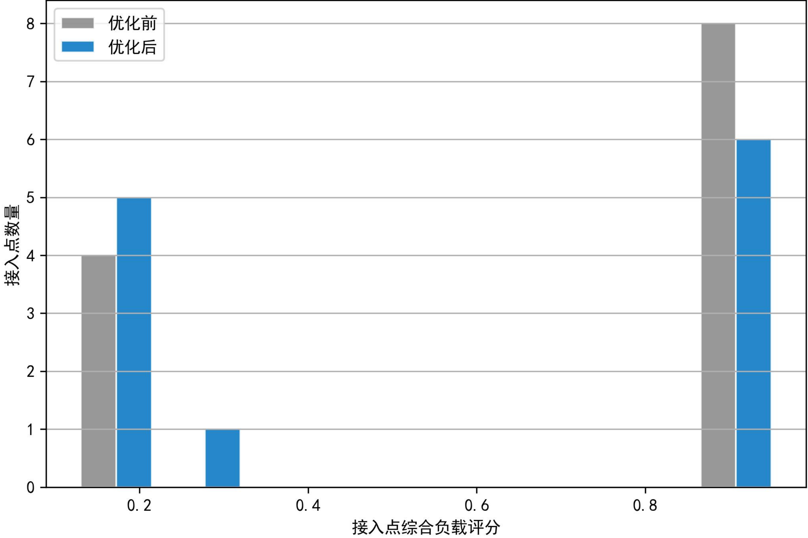
高峰时段 (19:00) 资源优化前后负载分布
