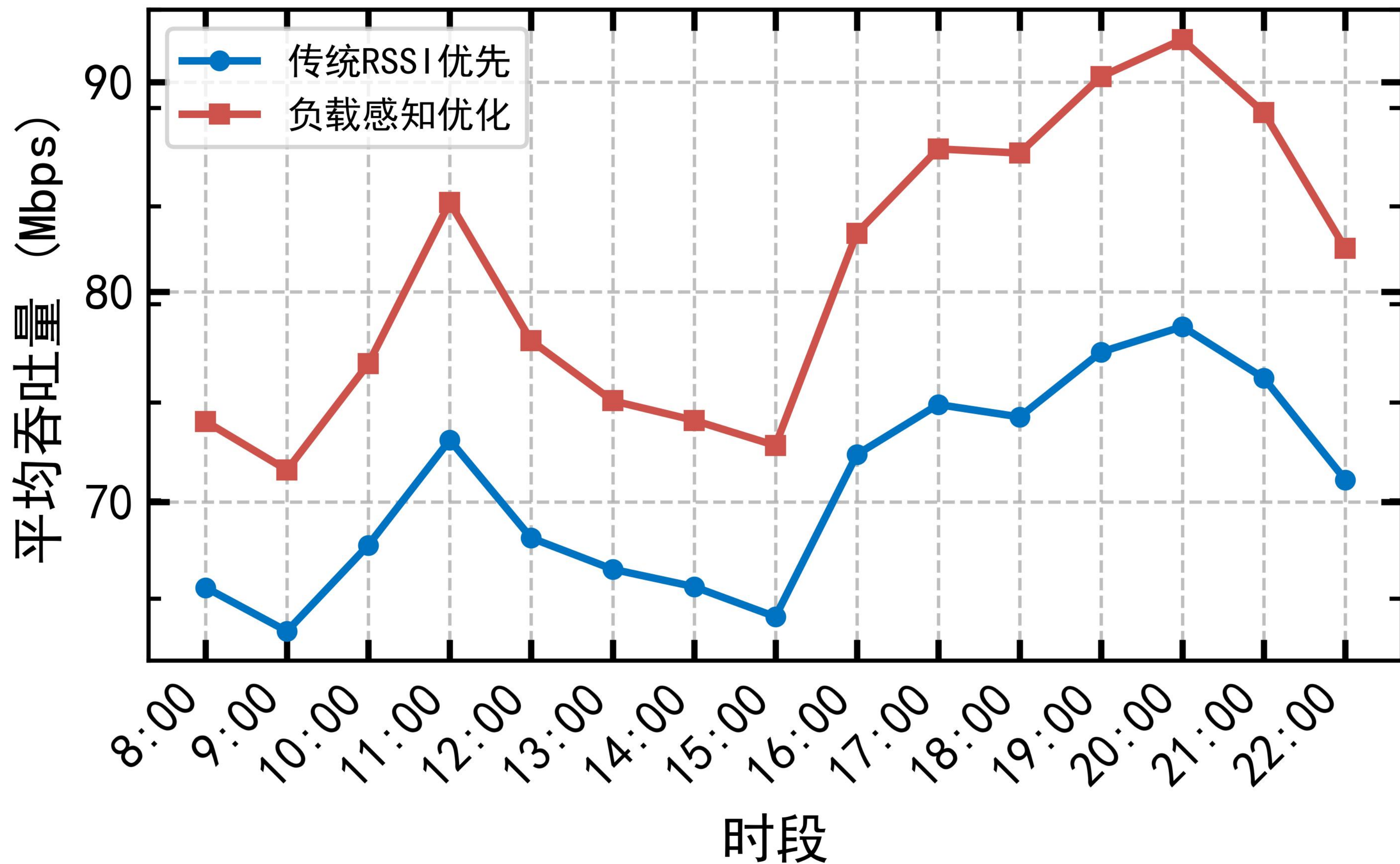
平均吞吐量对比
