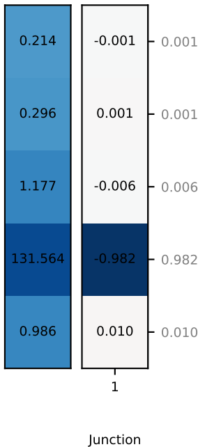
Shift (MHz)Participation
