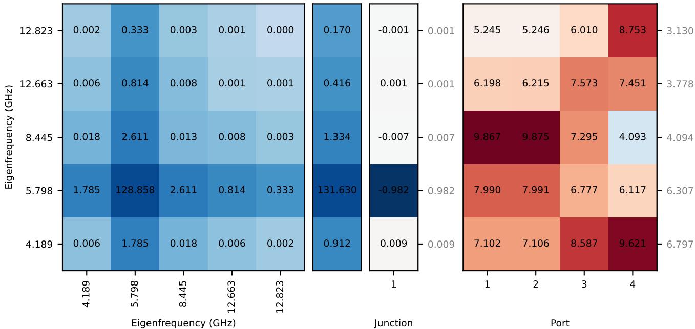
Kerr coupling (MHz)
