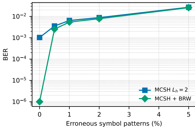
(d) Hopping-pattern desynchronization
