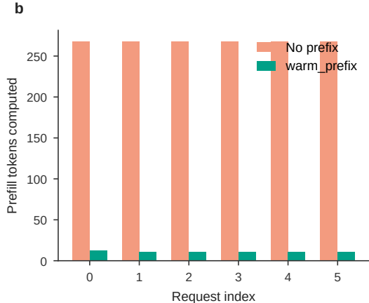
a: KV simulation (2048-token system prompt). b: gpt2 llmtr_paged E2E prefill savings.
