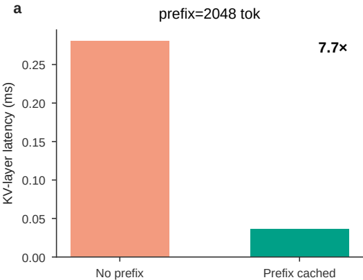
a: KV simulation (2048-token system prompt). b: gpt2 llmtr_paged E2E prefill savings.
