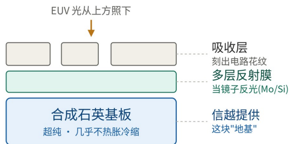
图 3 EUV 掩模基板的横截面：合成石英基板 + 多层反射膜 + 吸收层
