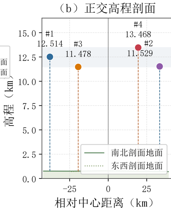
图1 问题三四个残骸的水平投影与高程剖面
