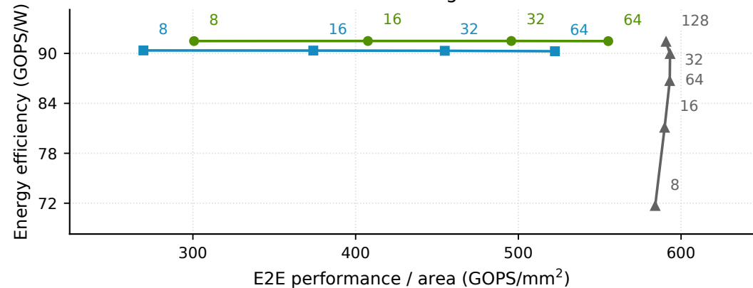
EDP tiling
