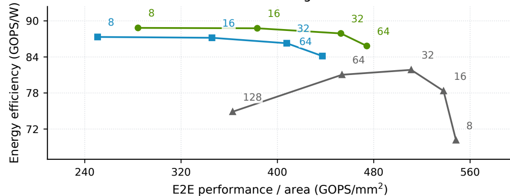
EDP tiling
