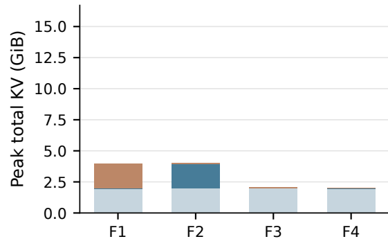
4K context
