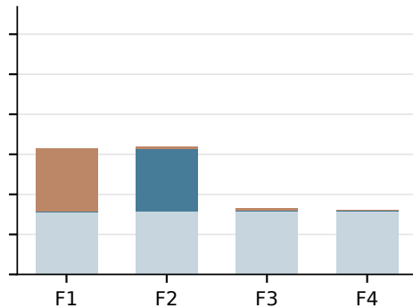
8K context
