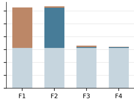
16K context
