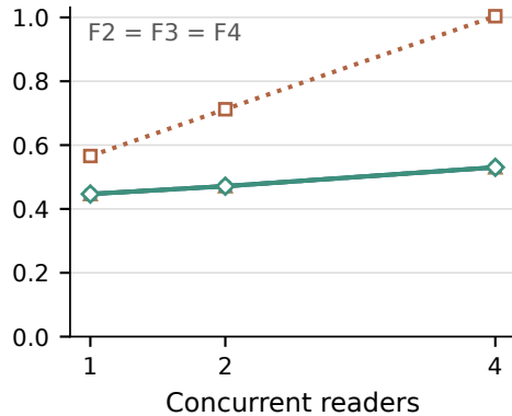
TBT
