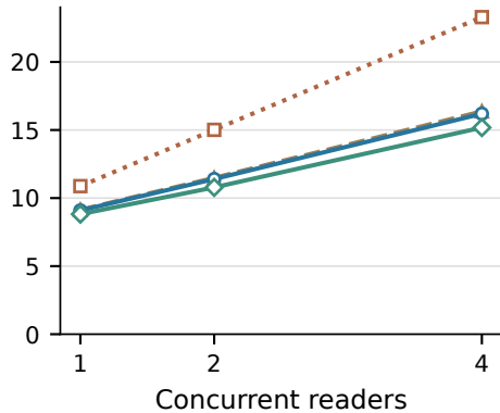
E2E
