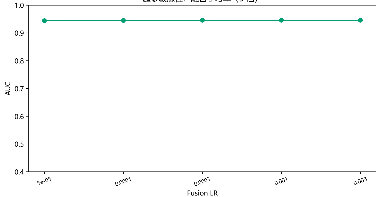
超参敏感性：融合学习率 (5 档)
