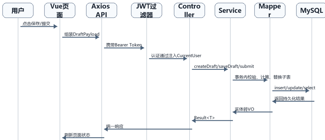
程序时序图：保存草稿与提交
