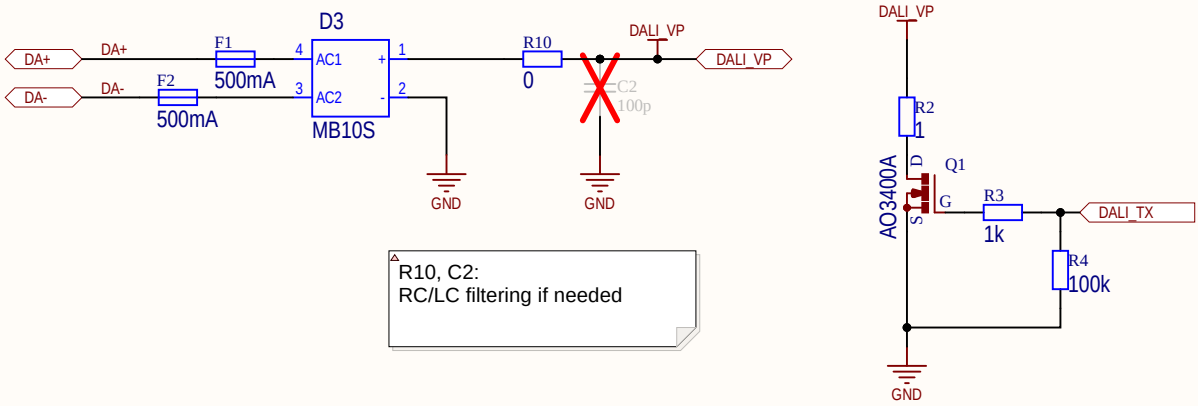
DALI Sender
