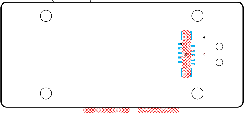
Bottom SMD (Scale 2:1)
