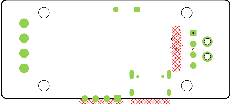
Bottom THT (Scale 2:1)
