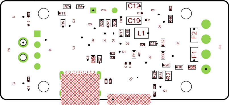
Top THT (Scale 2:1)
