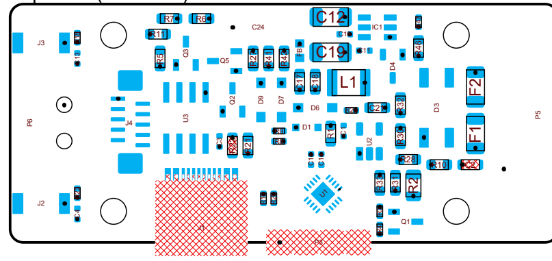
Top SMD (Scale 2:1)
