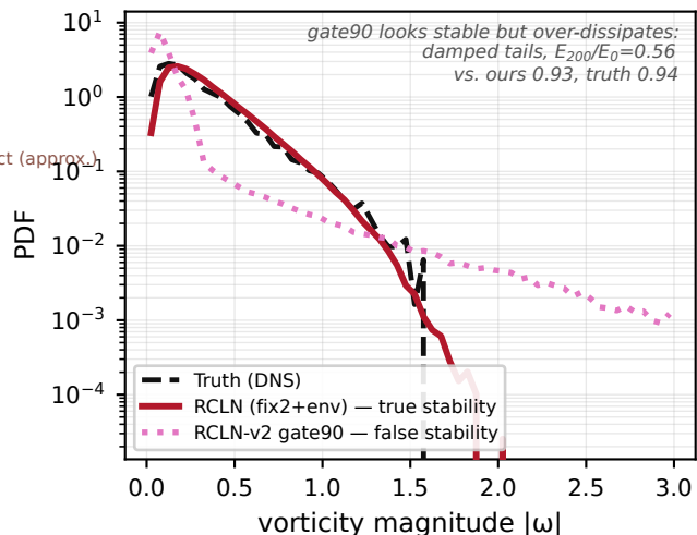
(d) Vorticity PDF @ k=200 : false vs. true stability
