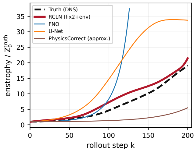
(d) Enstrophy, small-scale content
