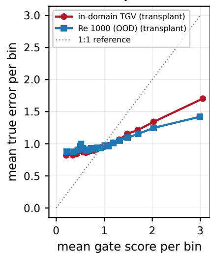
(d) Reliability (score vs. error)
