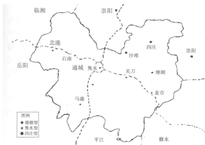
图 1 通城方言通摄阳声韵韵尾类型
