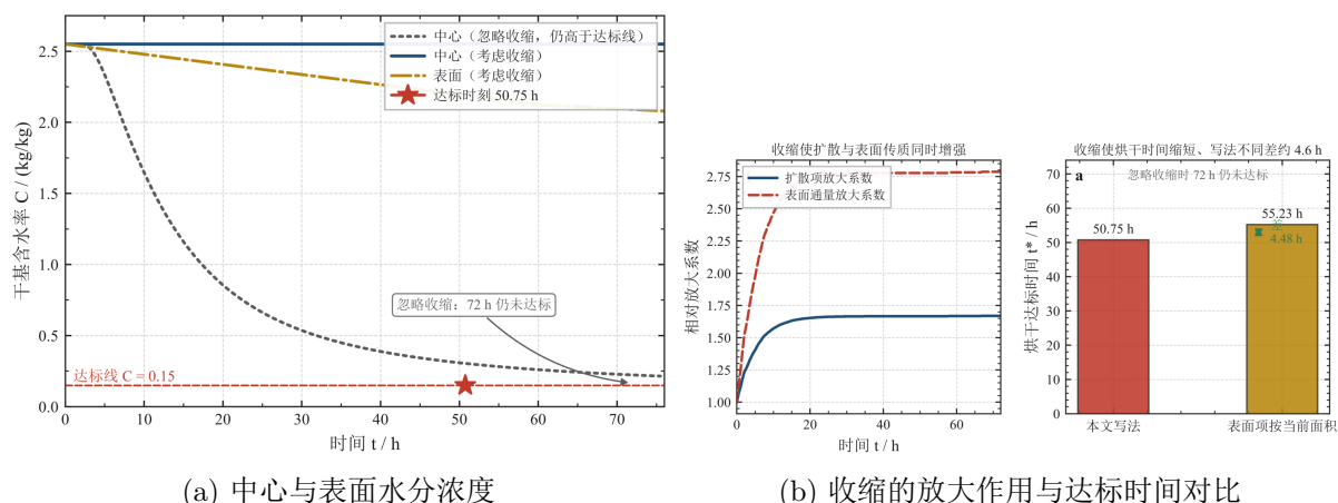
图 6 考虑收缩与忽略收缩时烘干过程的对比
