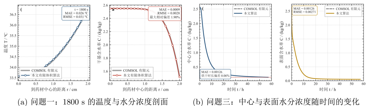
图 7 有限体积解与有限元仿真的对比（问题一、问题三）
