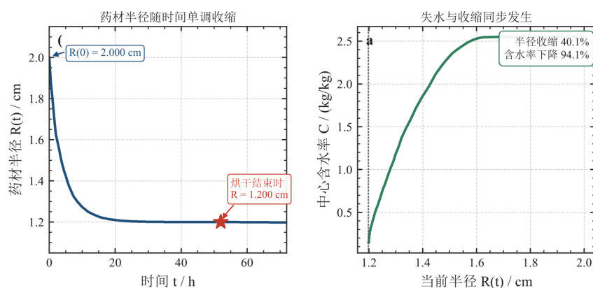
图 5 药材半径随时间的收缩规律及其与失水的同步性
