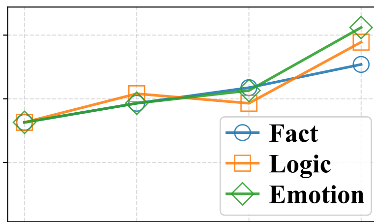
Weibo20
