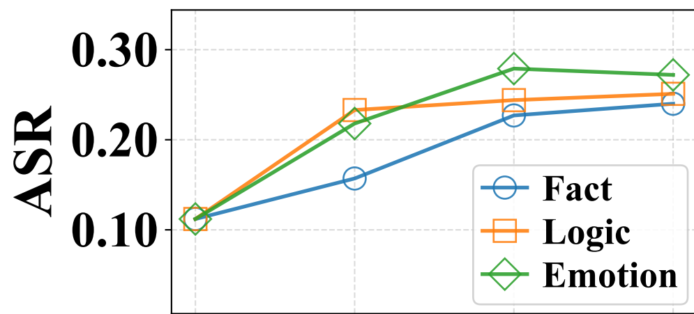
Weibo16
