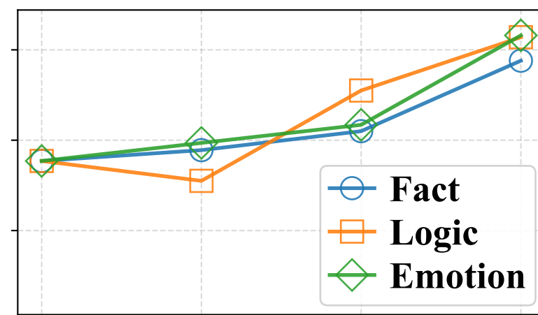
RumourEval
