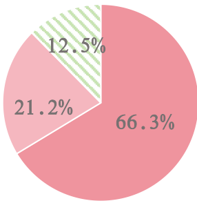
Qwen3-4B
