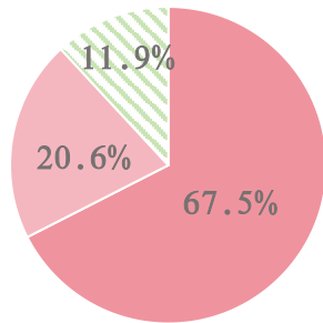
Qwen3-8B
