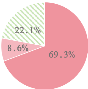
Llama3-8B
