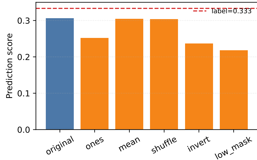
Prediction shift
