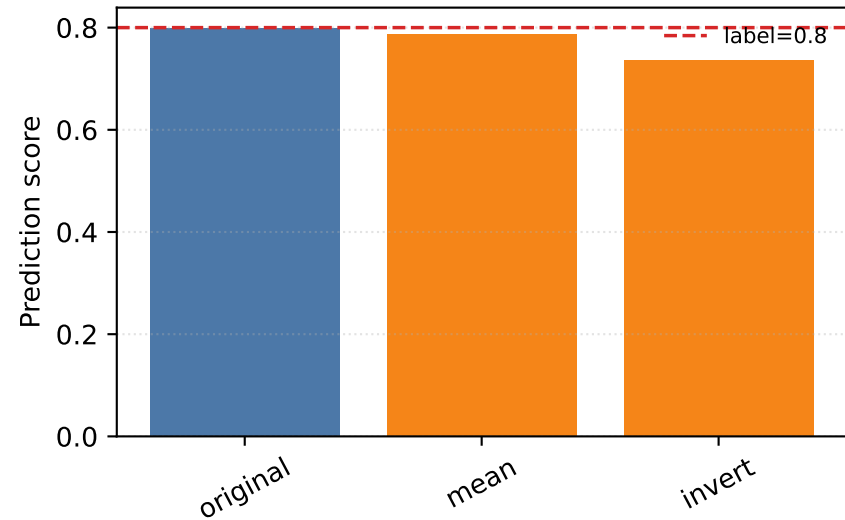
Prediction shift
