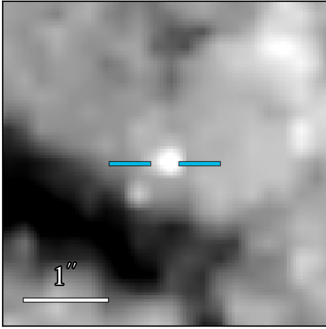
ACS F814W
