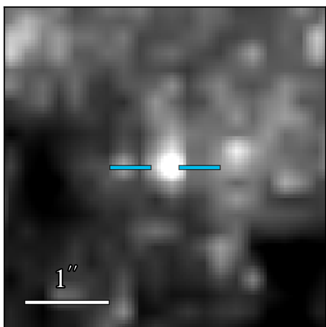
ACS F814W
