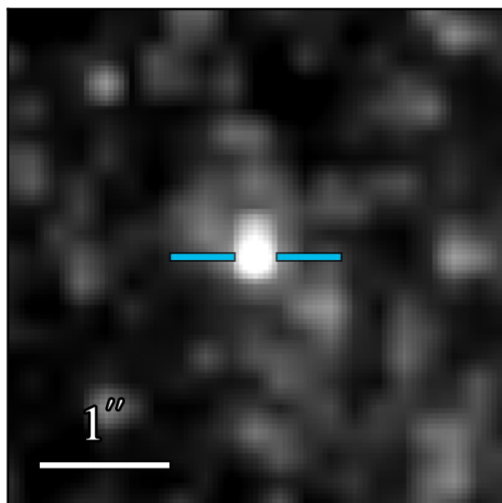
ACS F814W
