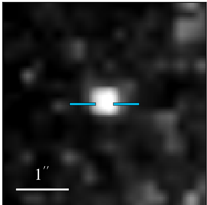
ACS F814W
