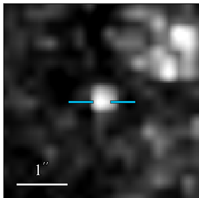
ACS F814W
