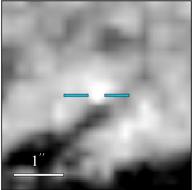
ACS F814W
