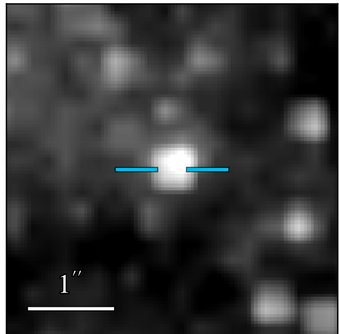
ACS F814W
