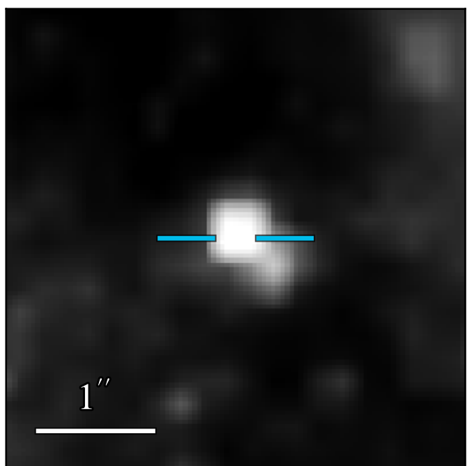
ACS F814W
