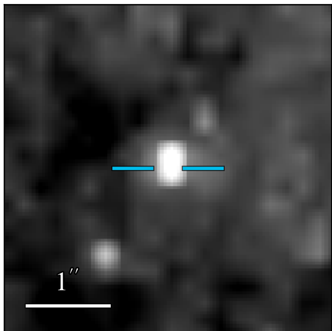
ACS F814W
