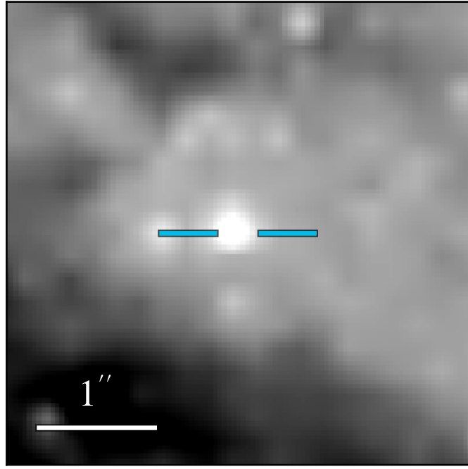
ACS F814W
