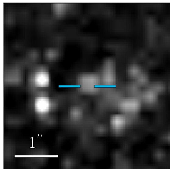
ACS F814W
