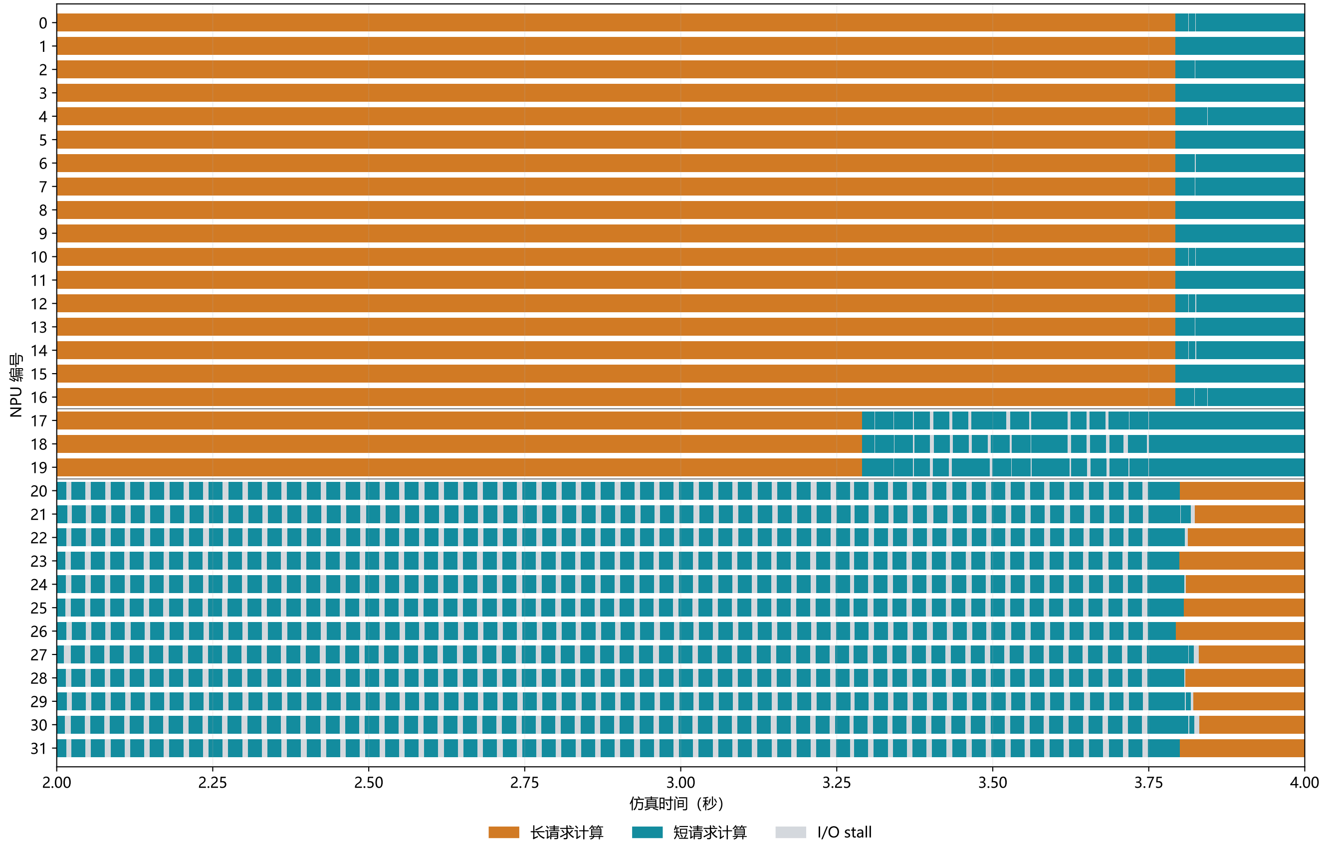
每卡长短混合：Baseline 的计算与 I/O 等待 32 NPU · 6 SSU · warm [2,4)s · 平均利用率 89.57%
