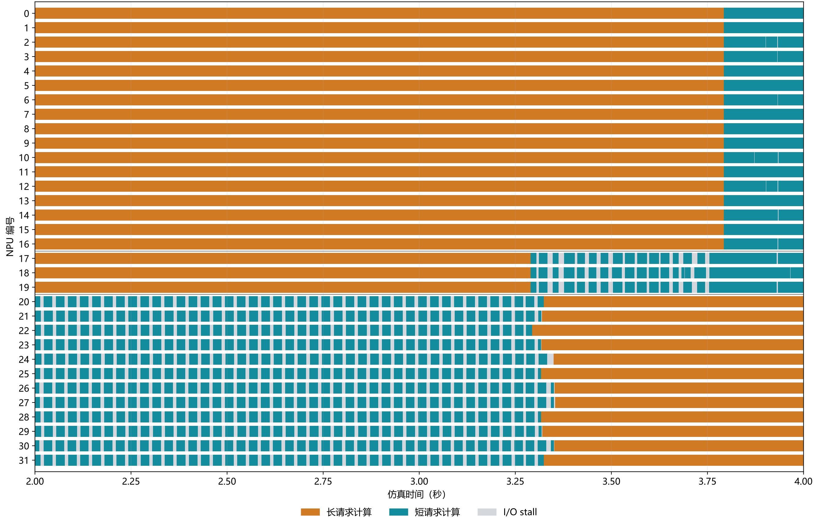
每卡长短混合：Baseline 的计算与 I/O 等待 32 NPU · 6 SSU · warm [2,4)s · 平均利用率 91.62%
