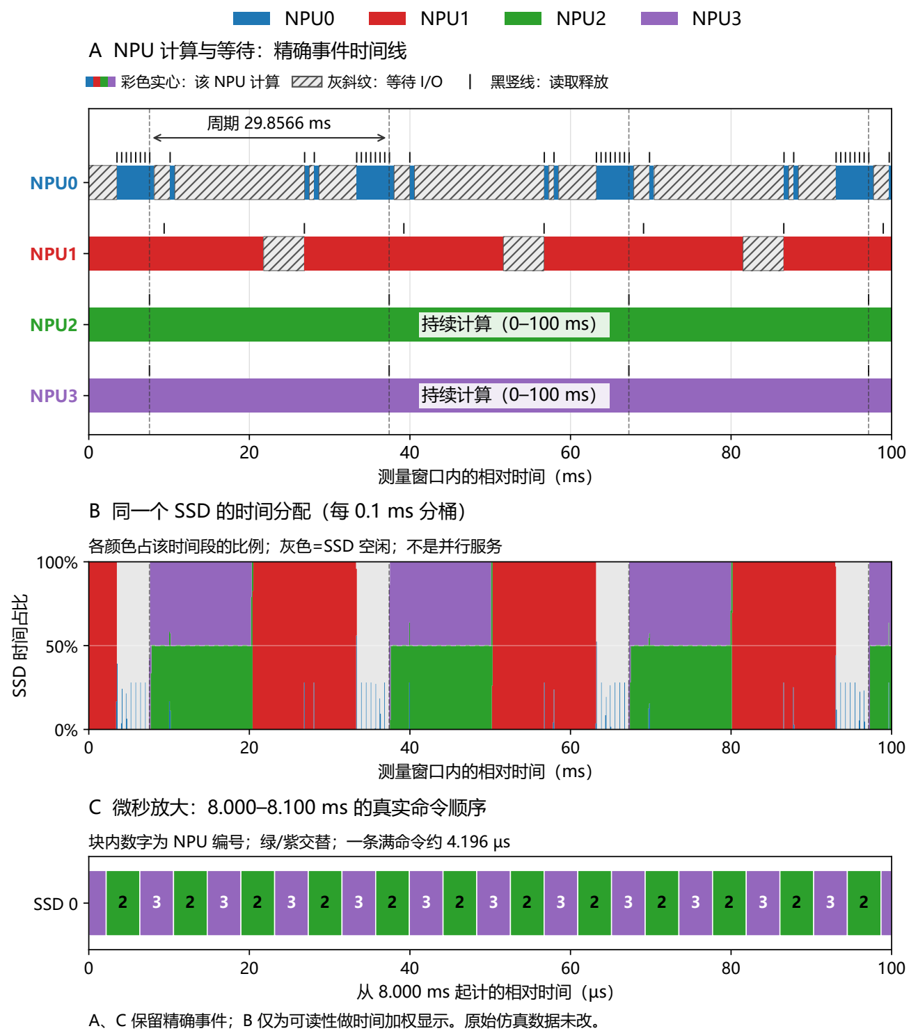
图 4： 同一 NPU 在三个子图中颜色一致。A 图的 NPU2 绿条、NPU3 紫条表示持续计算；B 图的分层色带是分桶后的时间比例，不是 SSD 同时并行服务；C 图给出精确的串行命令顺序。
