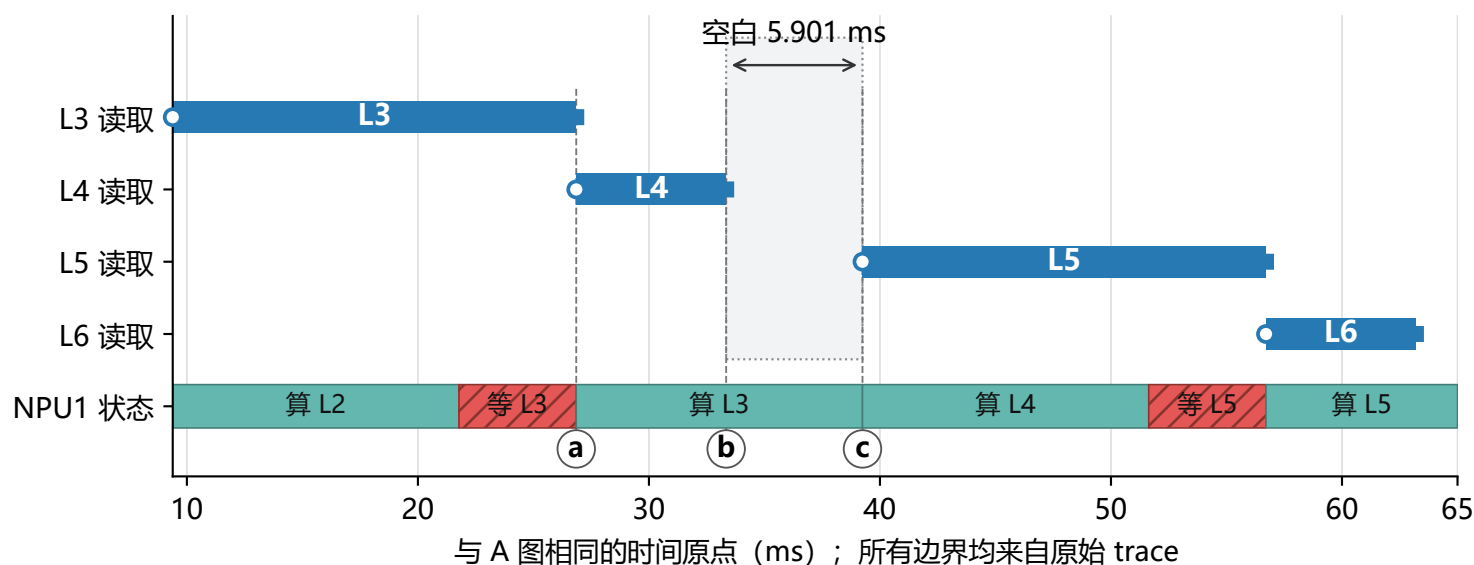
B NPU1 放大：分开看每一层的读取，再对照 NPU 状态
