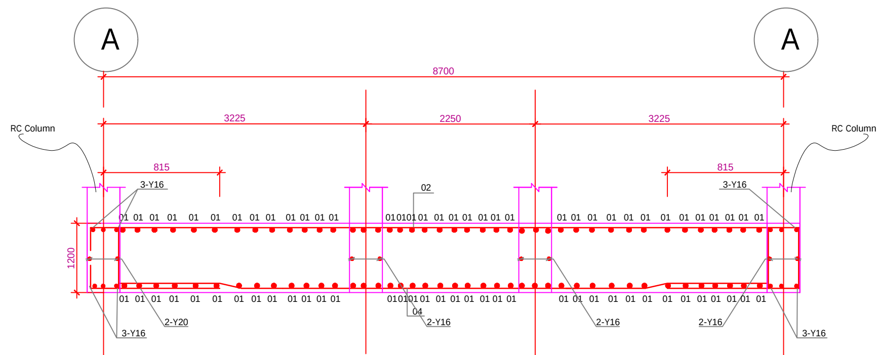
RAFT SLAB SECTION A-A.
