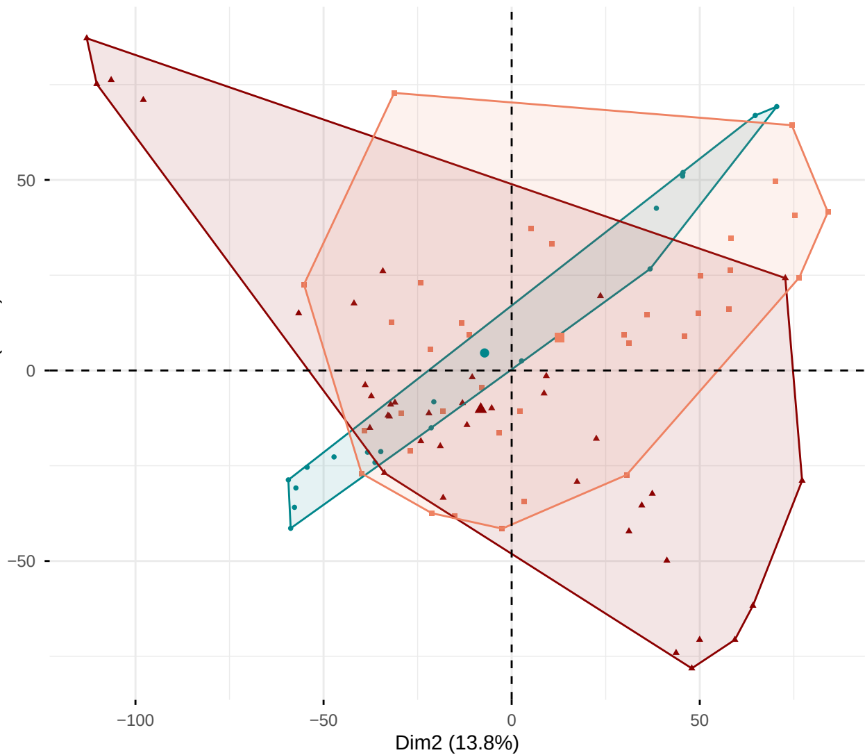
Individuals – PCA
