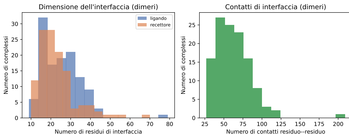
Figure 1: Distribuzione del numero di residui di interfaccia (sinistra) e del numero di contatti residuo-residuo (destra) sui complessi dimerici selezionati.
