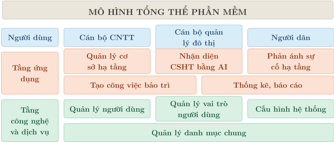
Hình 4.1 Mô hình tổng thể hệ thống
