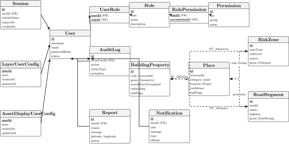
Hình 4.7 Sơ đồ Thực thể Kết hợp (ERD) mô tả cấu trúc cơ sở dữ liệu hệ thống.
