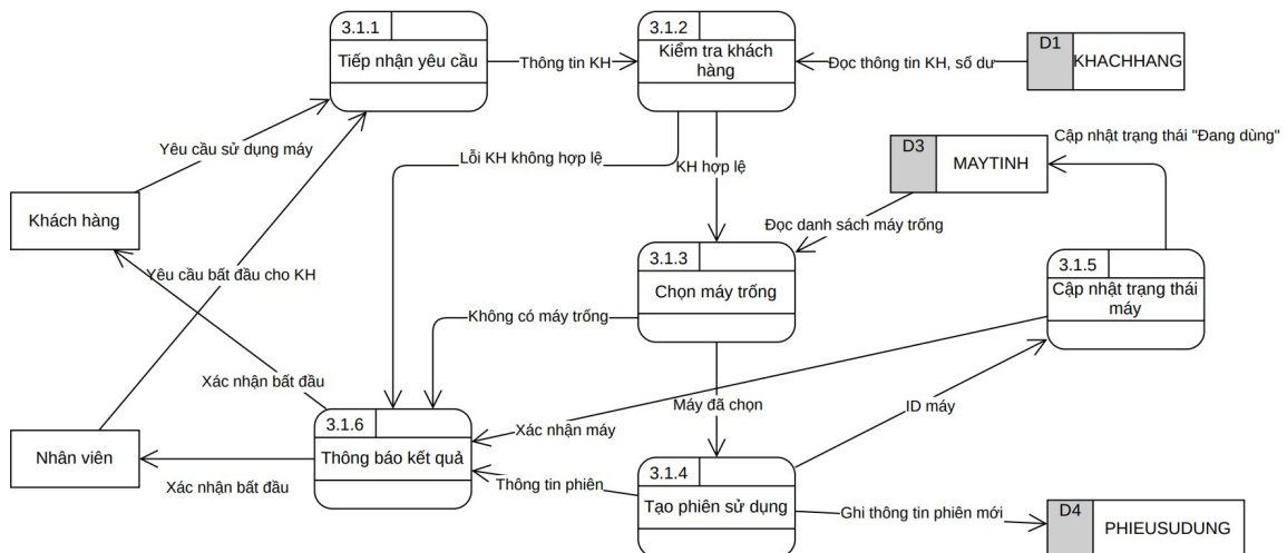
DFD Mức 3 - Tiến trình 3.1: Bắt đầu phiên
