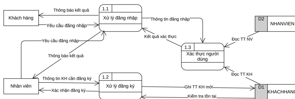
DFD Mức 2 – Quản lý tài khoản
