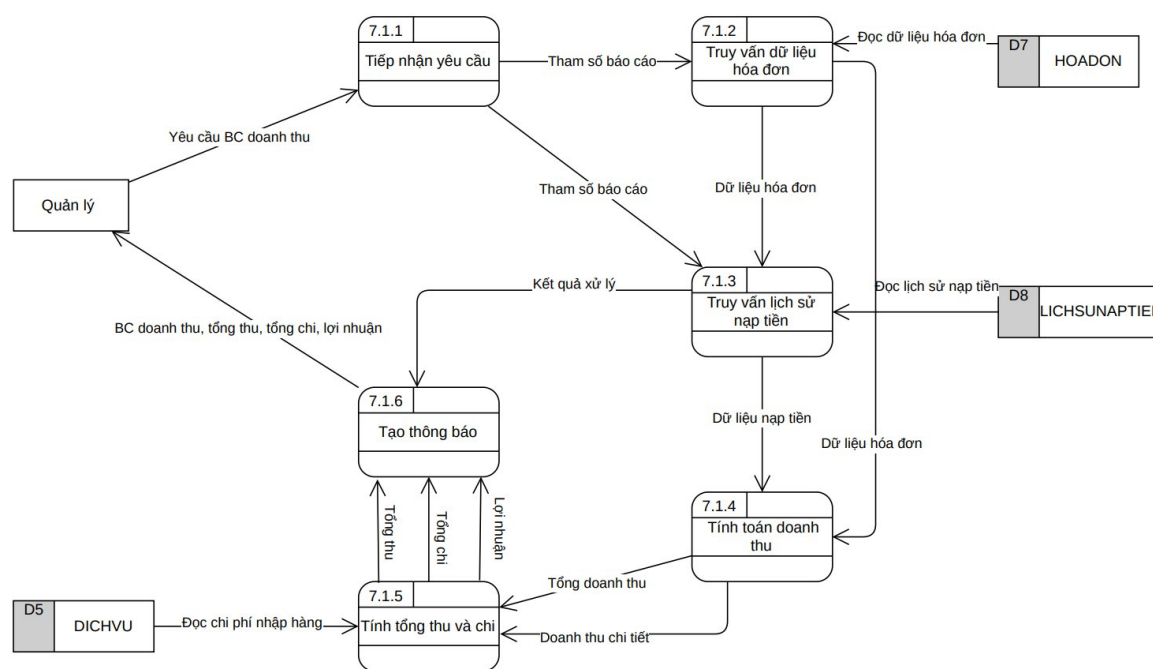
DFD Mức 3 - Tiến trình 7.1: Báo cáo doanh thu
