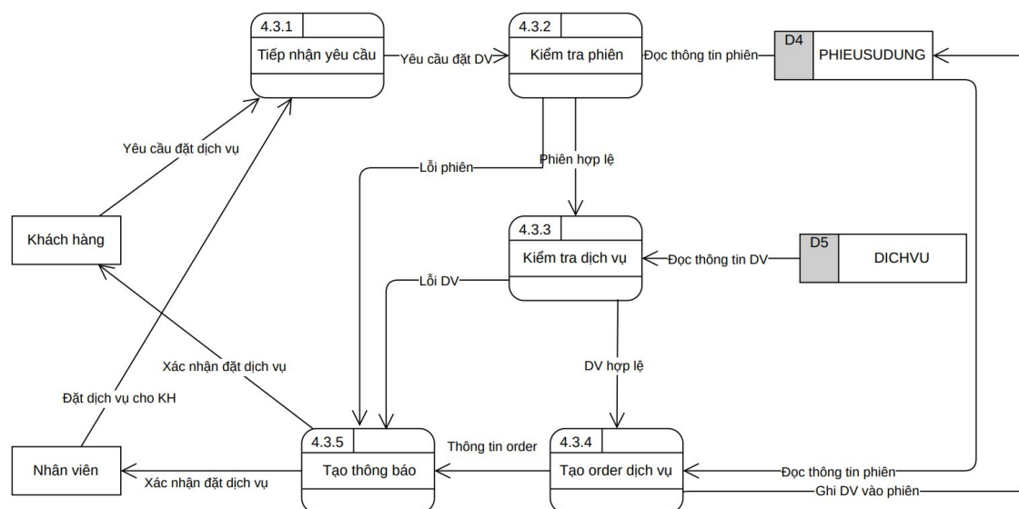
DFD Mức 3 - Tiến trình 4.3: Đặt dịch vụ trong phiên
