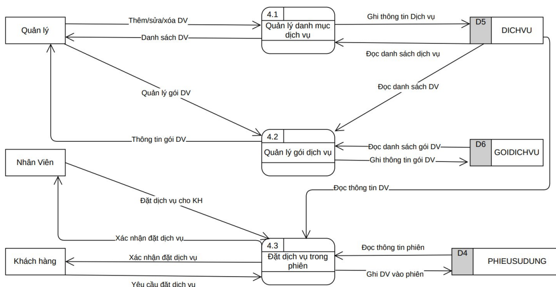
DFD Mức 2 – Quản lý dịch vụ
