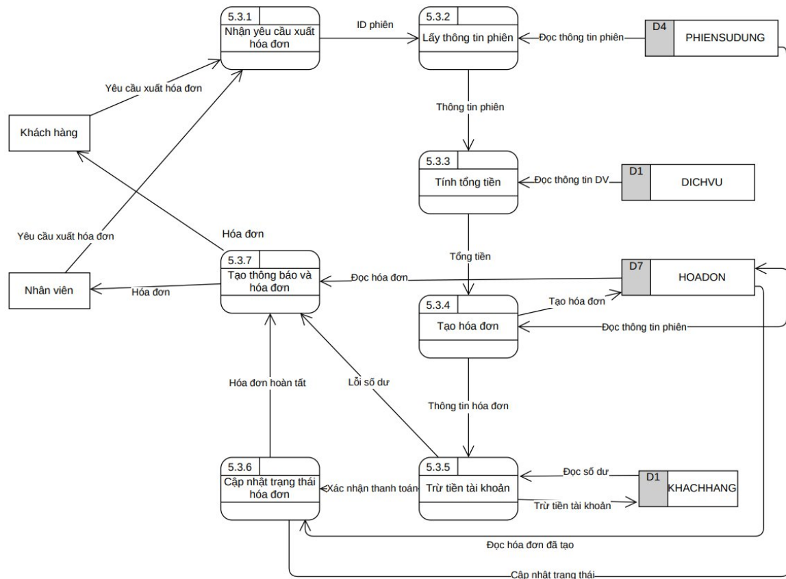
DFD Mức 3 - Tiến trình 5.3: Xuất hóa đơn
