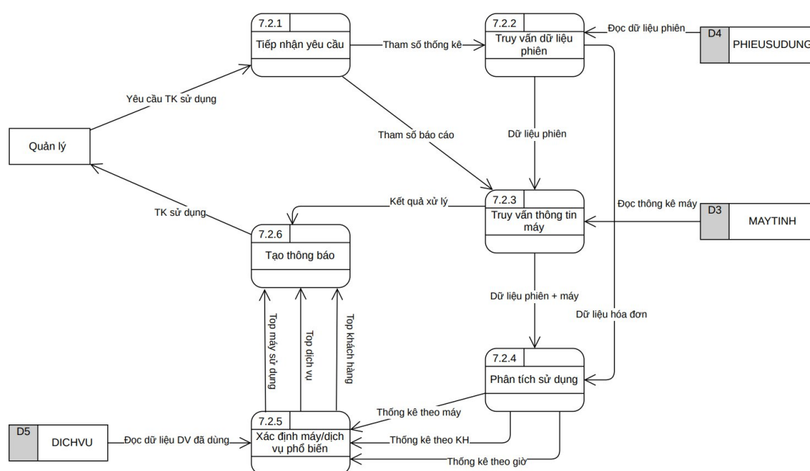
DFD Mức 3 - Tiến trình .2: Thống kê sử dụng
