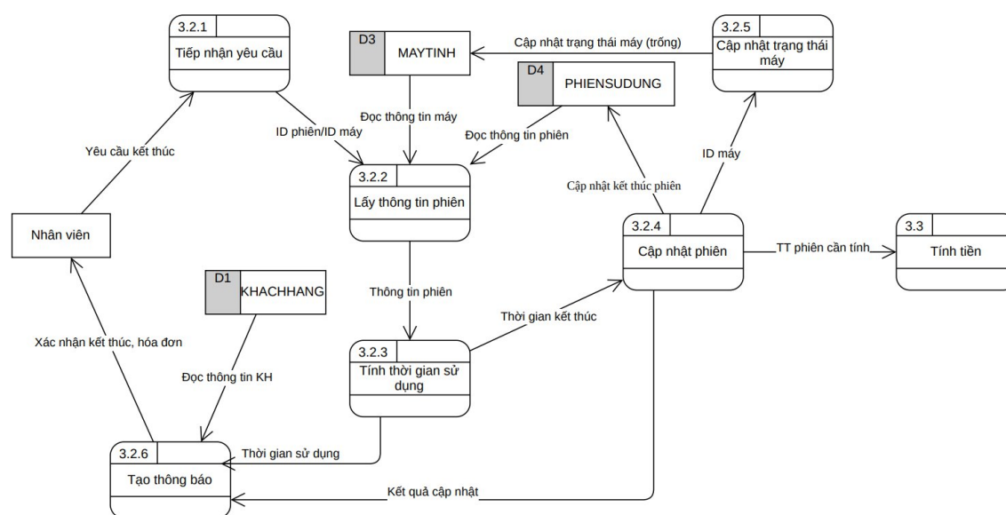
DFD Mức 3 - Tiến trình 3.2: Kết thúc phiên
