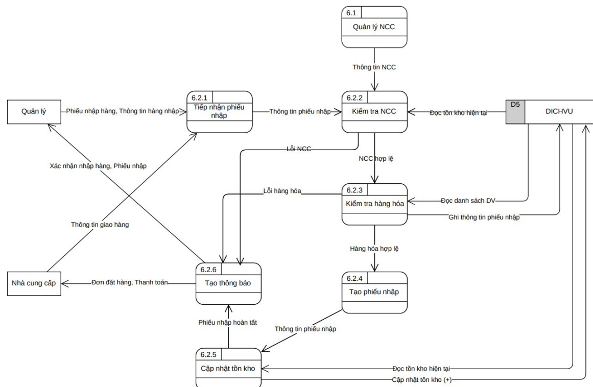
DFD Mức 3 - Tiến trình 6.2: Nhập hàng
