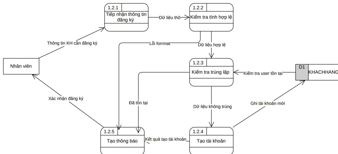
DFD Mức 3 - Tiến trình 1.2: Xử lý đăng ký
