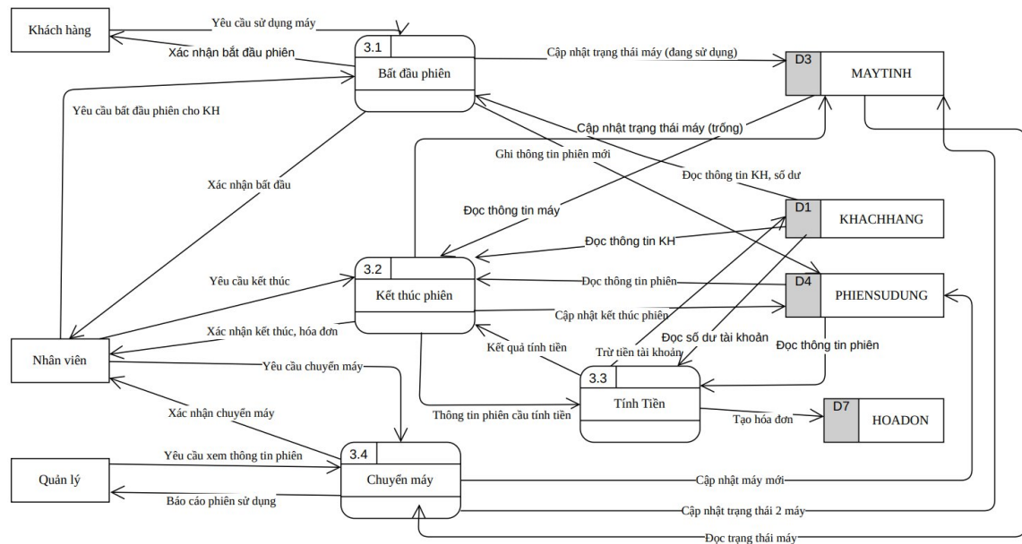
DFD Mức 2 – Quản lý phiên sử dụng
