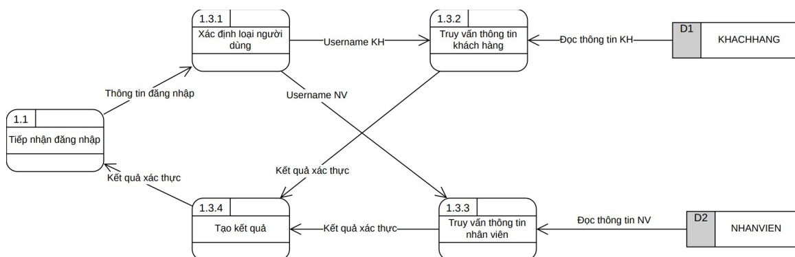
DFD Mức 3 - Tiến trình 1.3: Xác thực người dùng
