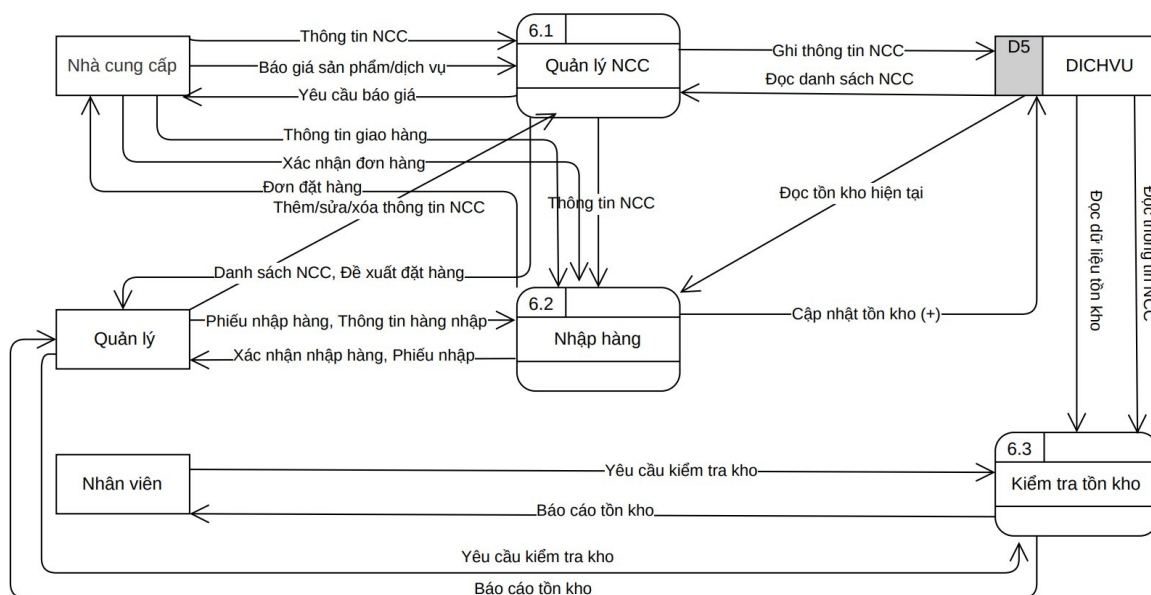
DFD Mức 2 – Quản lý kho hàng
