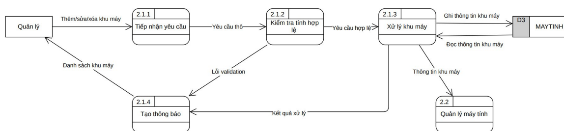
DFD Mức 3 - Tiến trình 2.1: Quản lý khu máy
