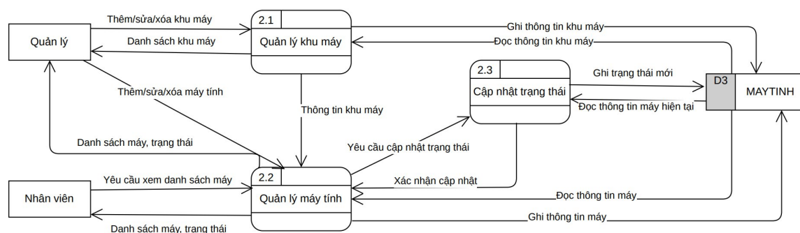
DFD Mức 2 – Quản lý máy và khu máy
