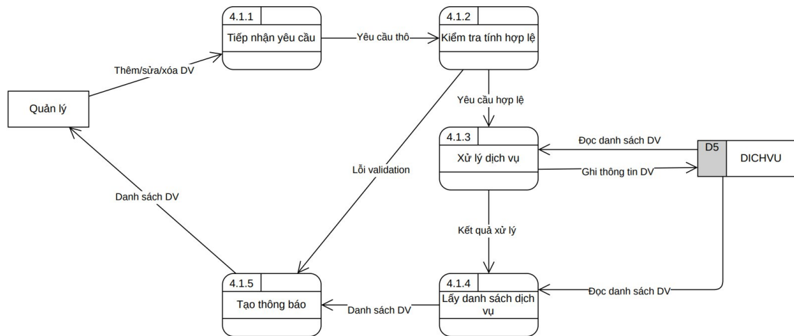
DFD Mức 3 - Tiến trình 4.1: Quản lý danh mục dịch vụ
