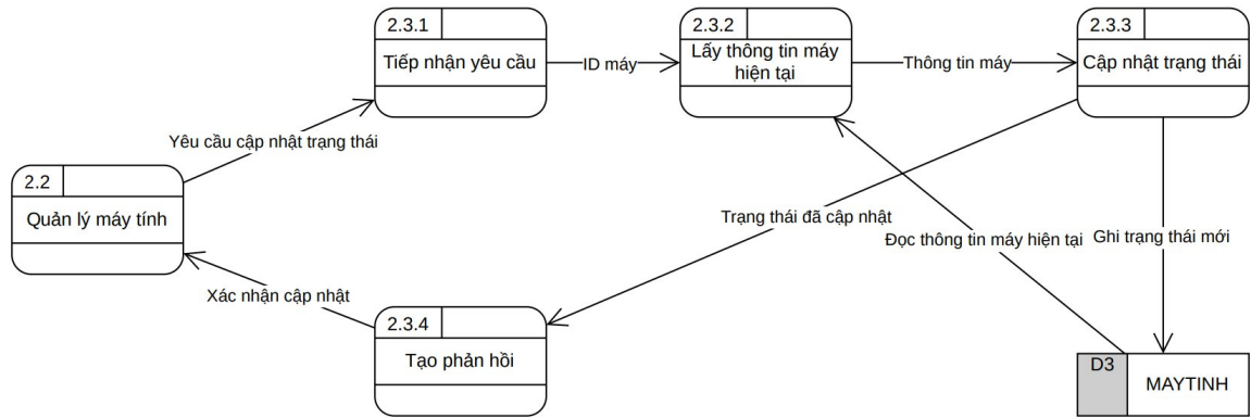
DFD Mức 3 - Tiến trình 2.3: Cập nhật trạng thái máy
