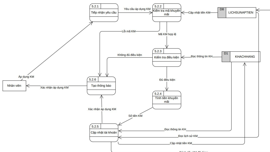
DFD Mức 3 - Tiến trình 5.2: Áp dụng khuyến mãi
