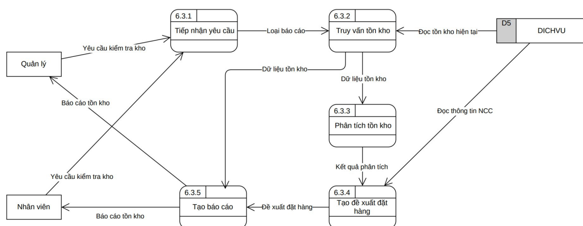
DFD Mức 3 - Tiến trình 6.3: Kiểm tra tồn kho
