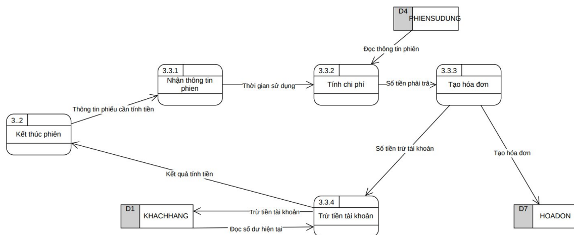
DFD Mức 3 - Tiến trình 3.3: Tính tiền
