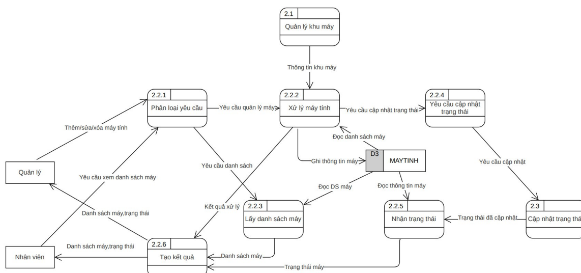
DFD Mức 3 - Tiến trình 2.2: Quản lý máy tính
