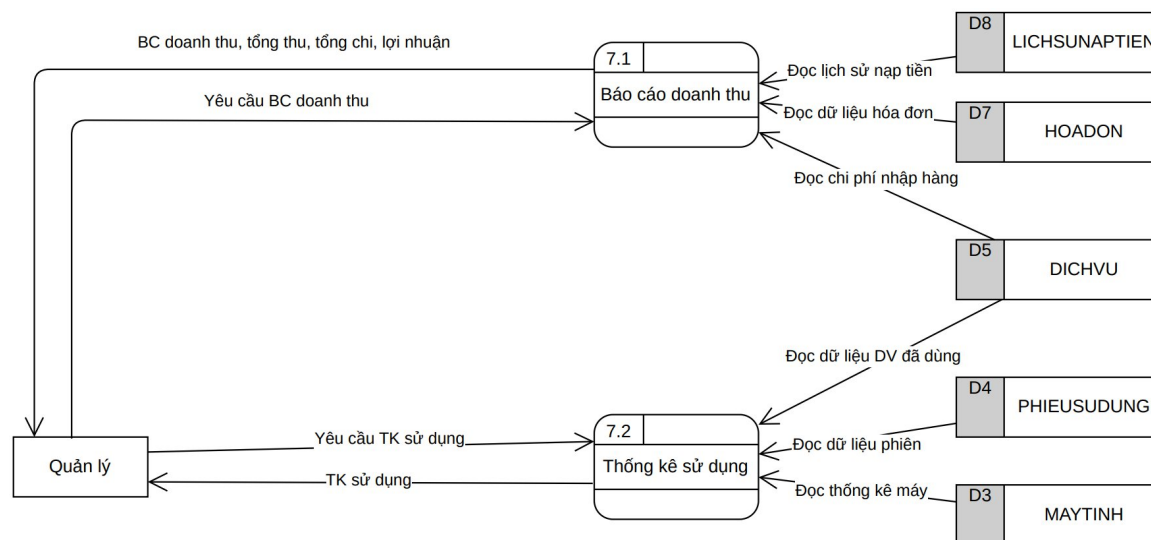
DFD Mức 2 – Báo cáo thống kê
