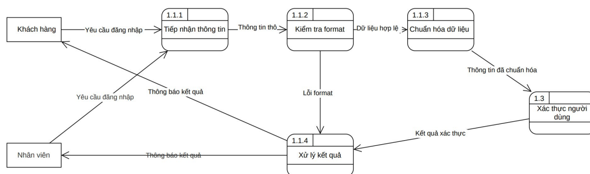
DFD Mức 3 - Tiến trình 1.1: Xử lý đăng nhập
