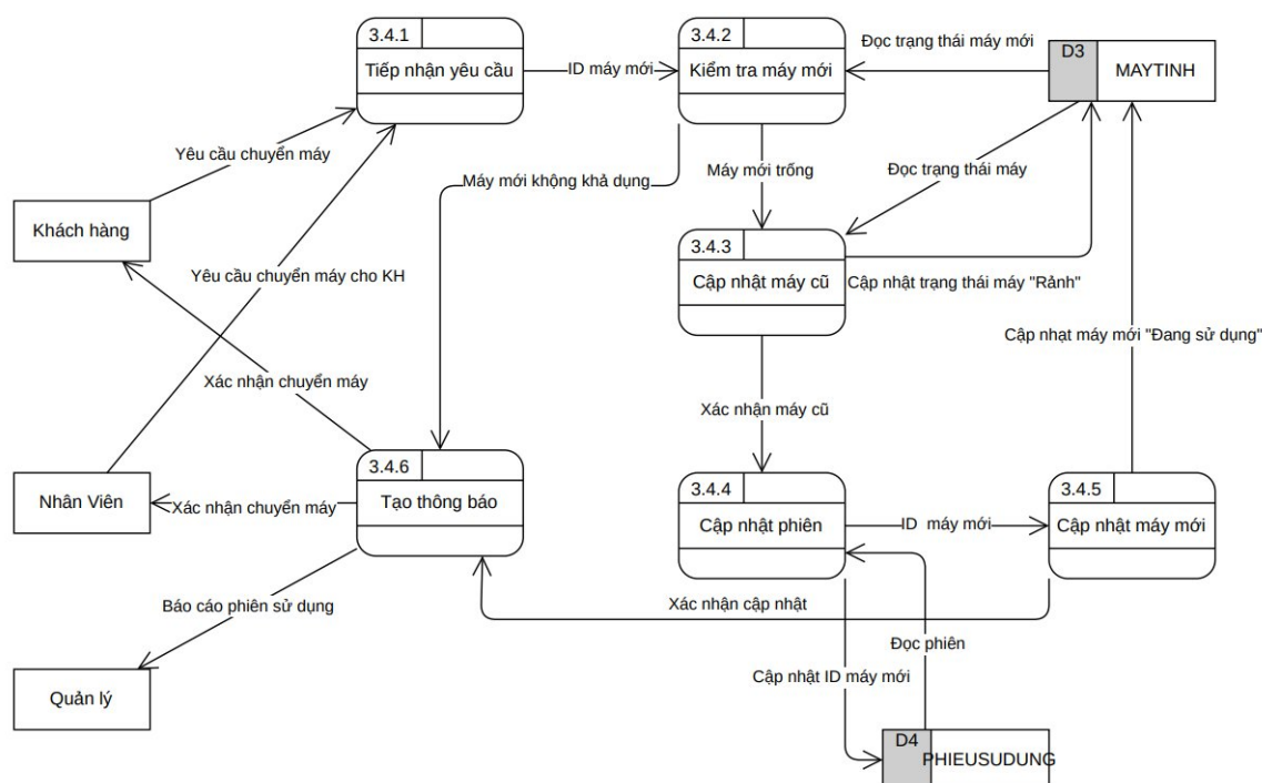
DFD Mức 3 - Tiến trình 3.4: Chuyển máy
