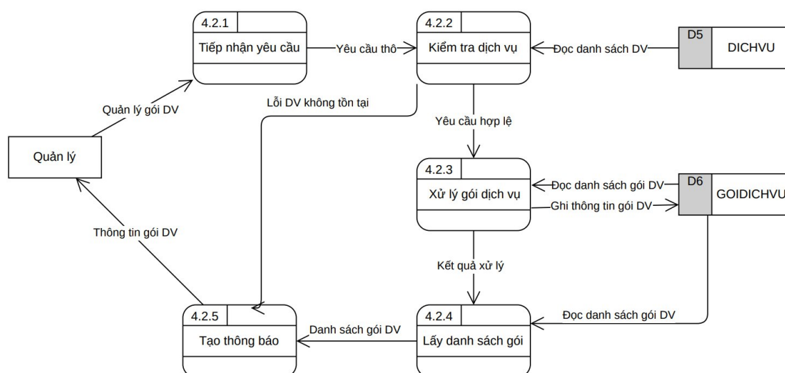
DFD Mức 3 - Tiến trình 4.2: Quản lý gói dịch vụ
