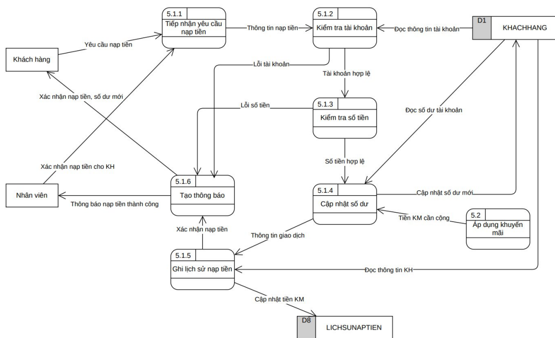
DFD Mức 3 - Tiến trình 5.1: Nạp tiền tài khoản
