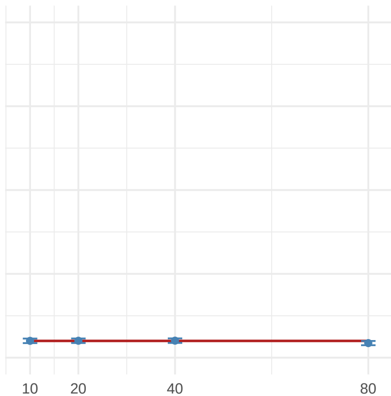
Null: Type I error
