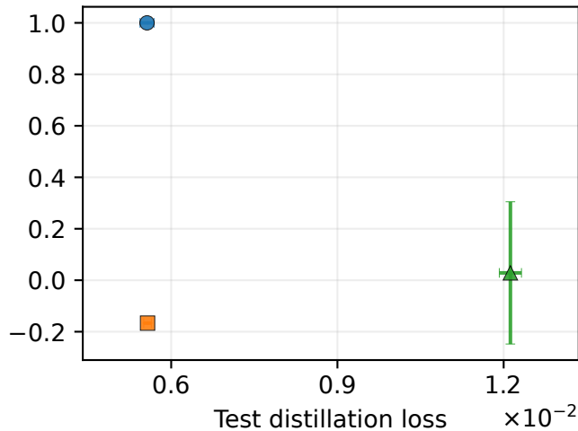
MLP
