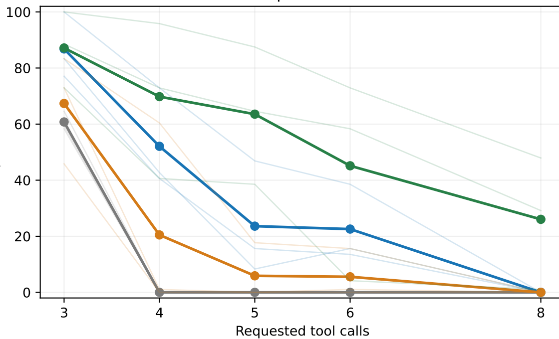
qwen7b
