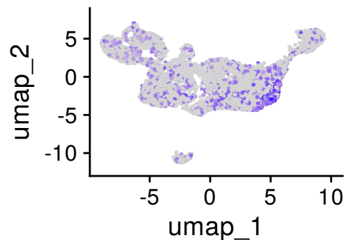
Il7r
