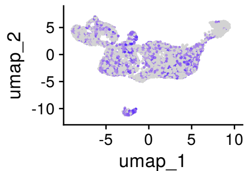
Il7r
