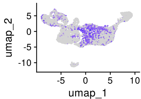
Lef1
