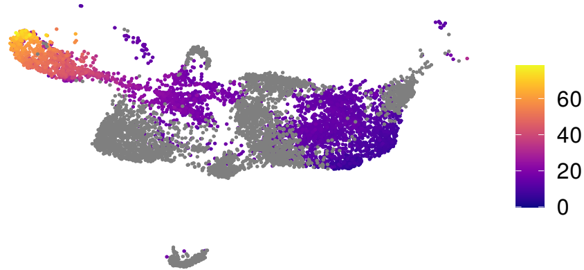
slingsPseudotime_7
