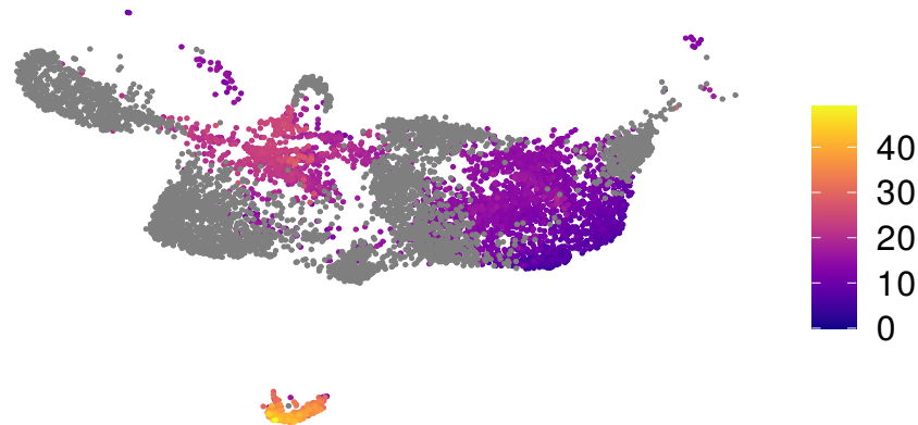
slingsPseudotime_5
